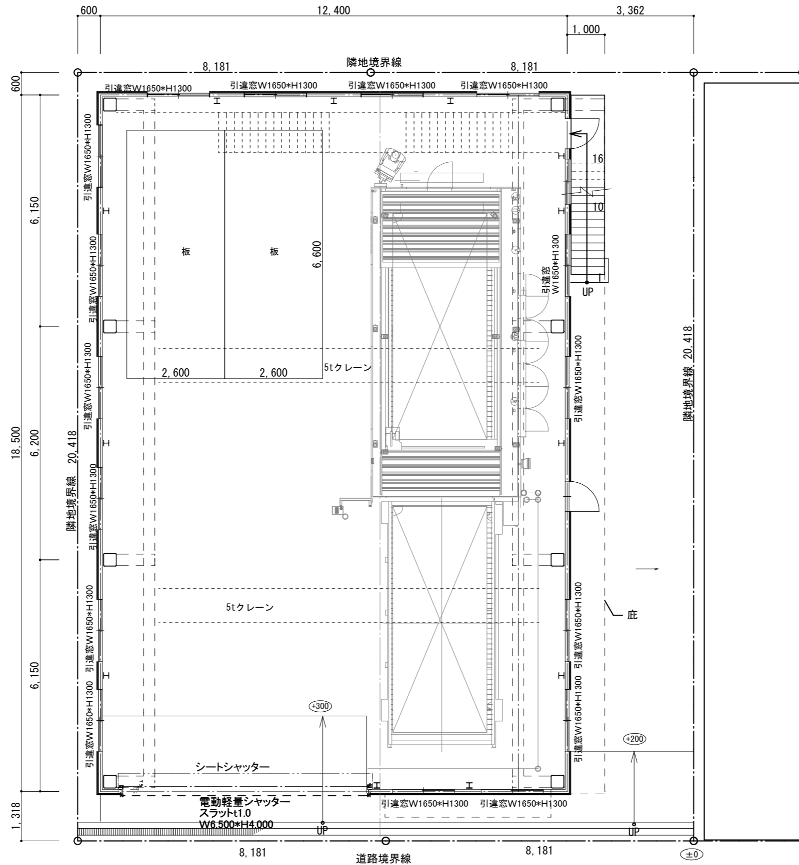
1階平面図 S=1/100 229.40 m 2
