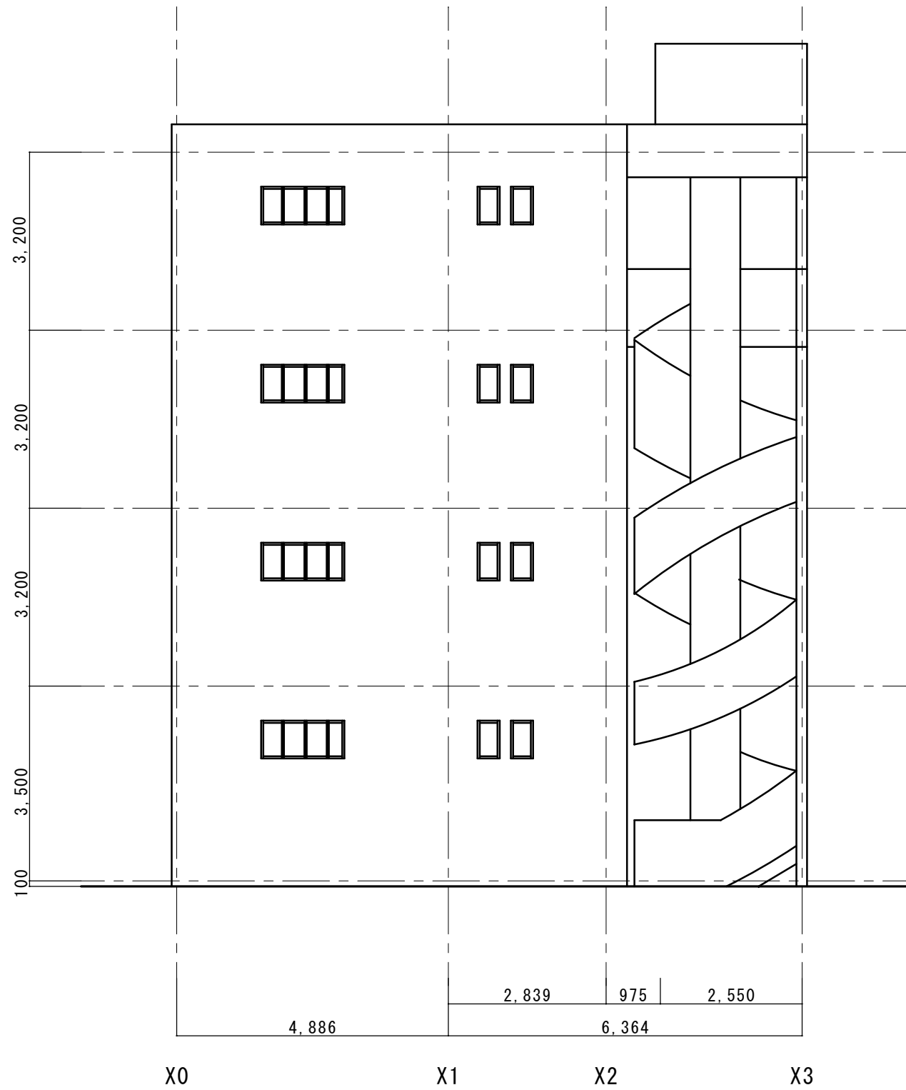
南立面图
