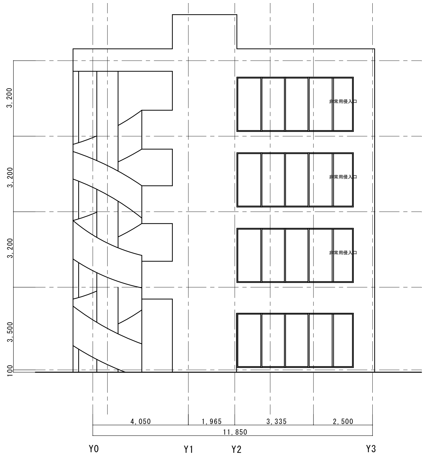
東立面图
