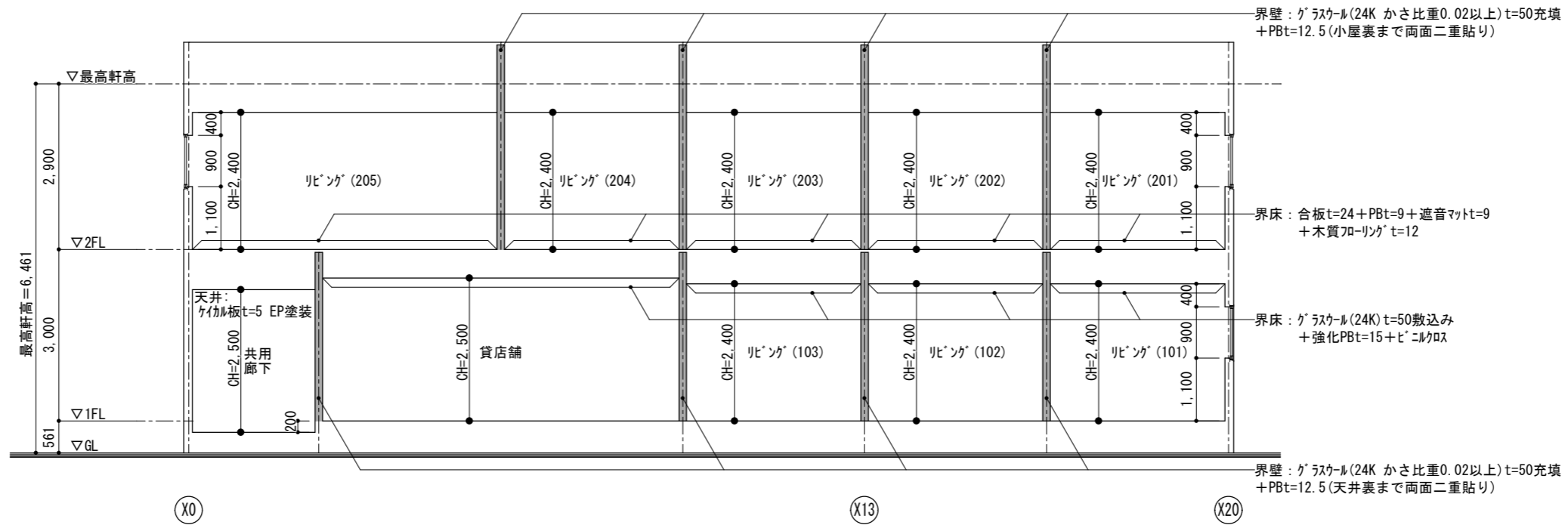
A-A' 断面図
