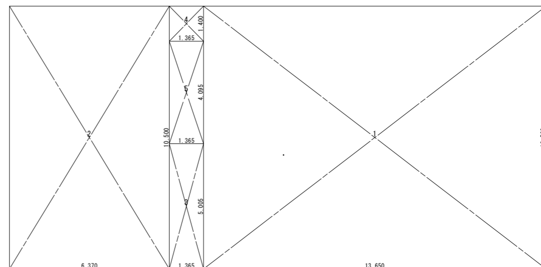
2階建物求積図 S=1/150
