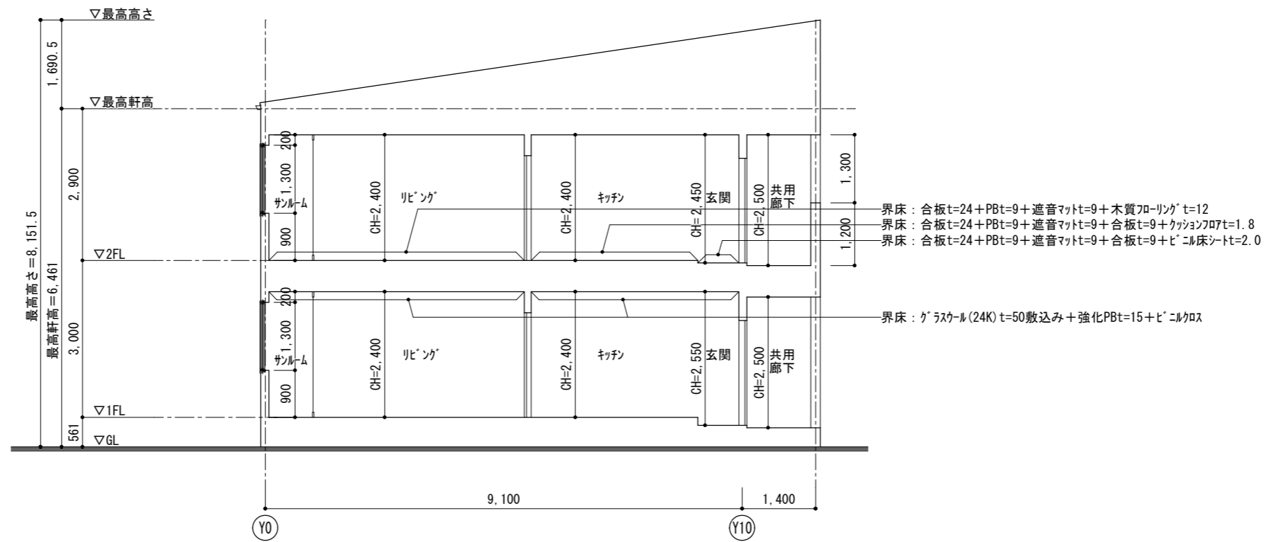
B-B' 断面図
