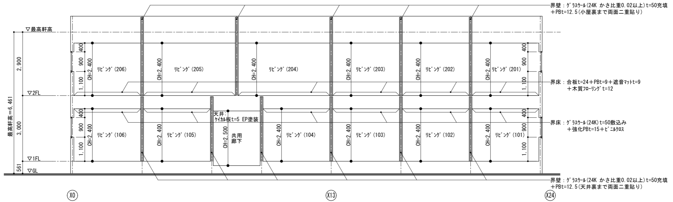
A-A' 断面図
