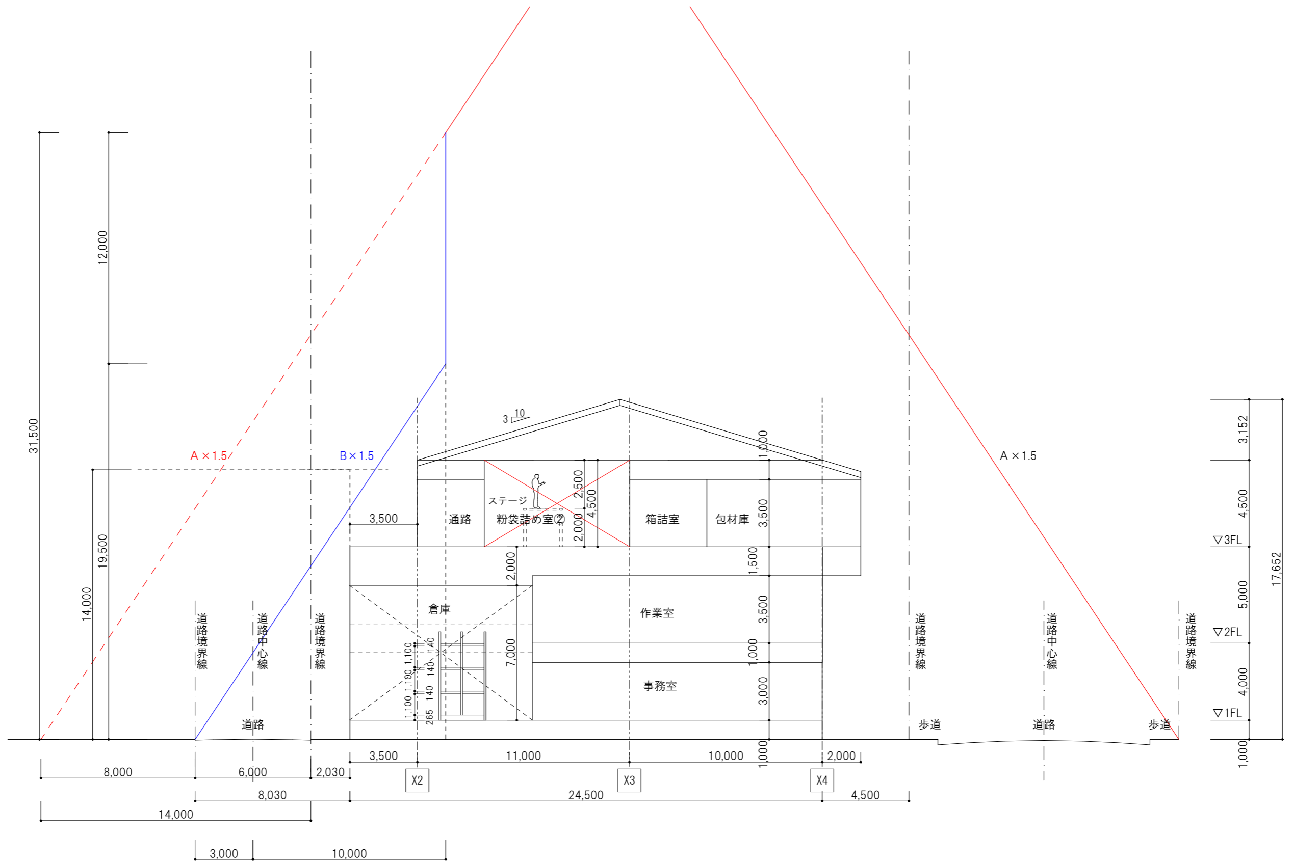
計画断面図 1:200
